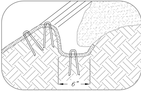
LONGITUDINAL ANCHOR TRENCH NTS
