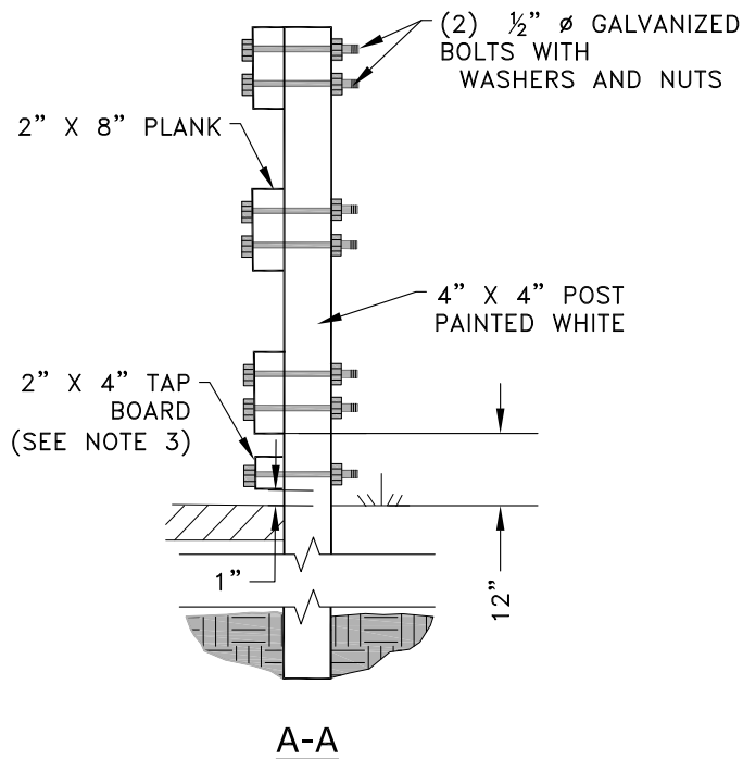
TYPE III BARRICADE
